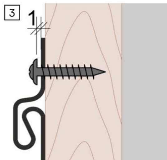
Рис. 2 Схема фиксации сайдинга Döcke.
