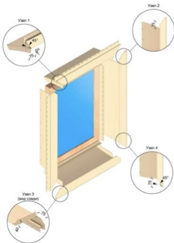
Рис. 15 Обрамление оконного проёма при помощи околооконного профиля.
