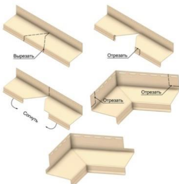
Рис. 6 Изготовление внутреннего углового элемента отлива Döcke.
