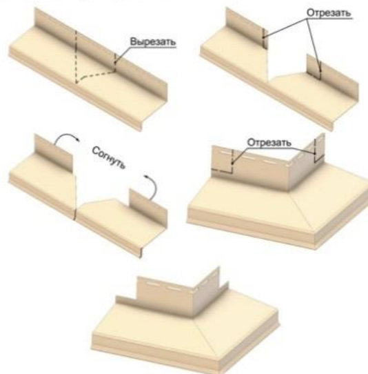
Рис. 4 Изготовление внешнего углового элемента отлива Döcke.
