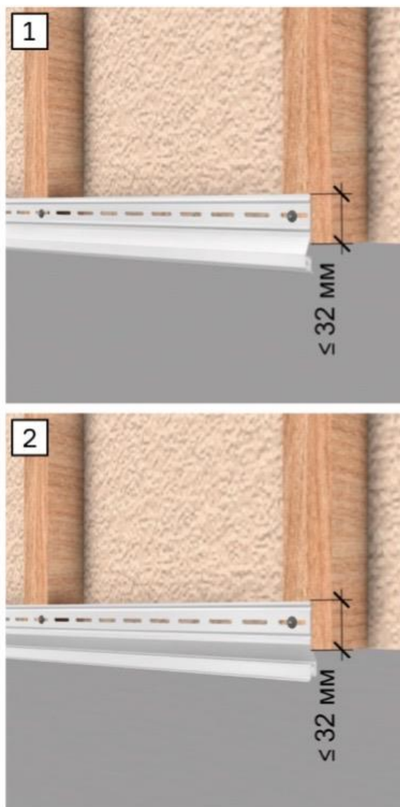
Рис. 12 Установка стартового профиля.
