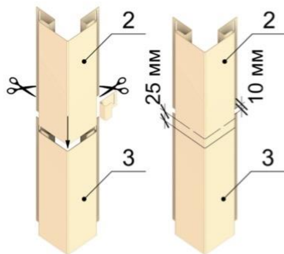
Рис. 8 Подрезка и стыковка наружных углов.
