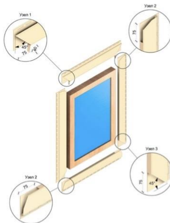
Рис. 13 Обрамление оконного проёма при помощи наличника 75 мм.
