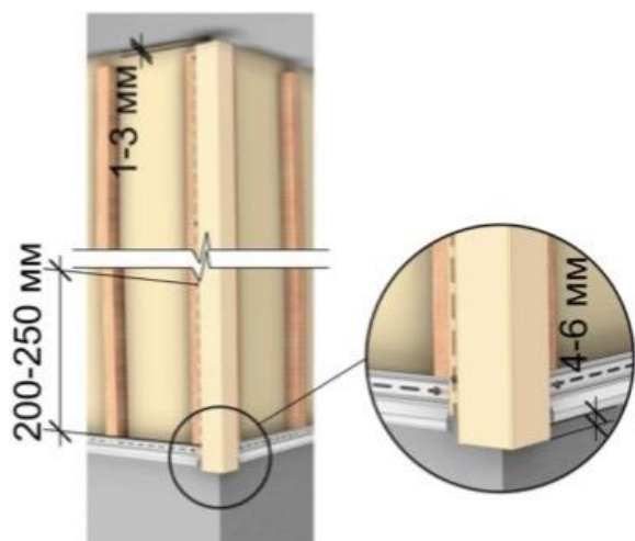
Рис. 7 Установка внешних углов.
