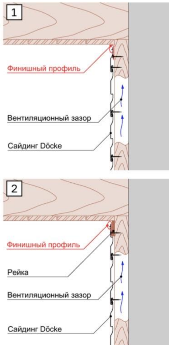
Рис. 25 Примыкание сайдинга Döcke к карнизному свесу при помощи финишного профиля.
