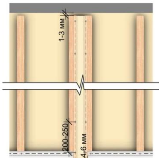
Рис. 10 Установка Н-профиля.
