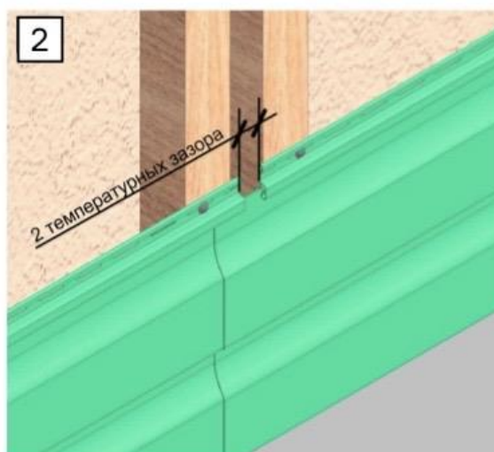
Рис. 23 Стыковка панелей горизонтального сайдинга Döcke внахлест.
