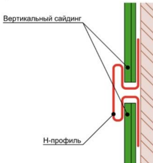
Рис. 31 Стыковка вертикального сайдинга по длине.
