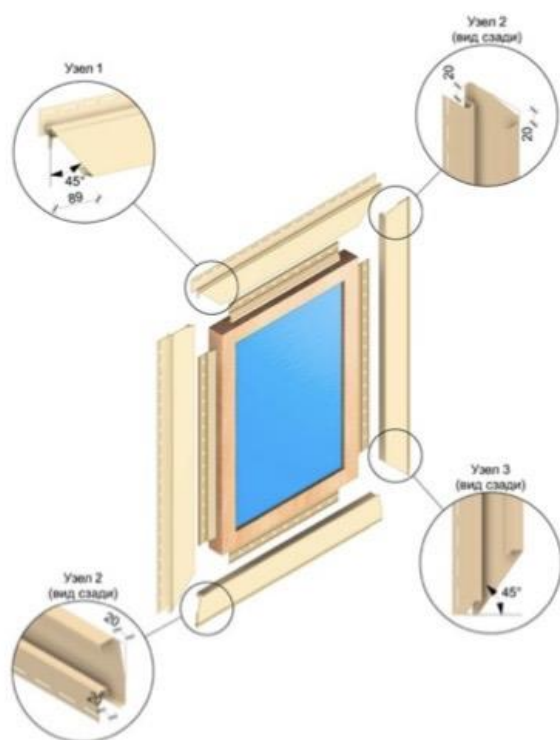
Рис. 14 Обрамление оконного проёма при помощи наличника 89 мм.
