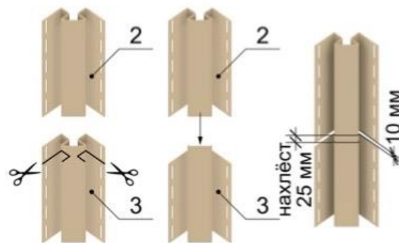
Рис. 9 Подрезка и стыковка внутренних углов.
