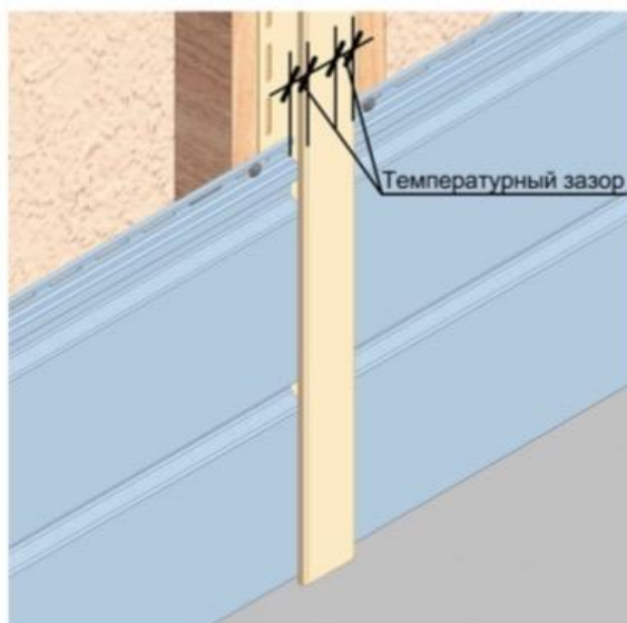
Рис. 22 Стыковка панелей горизонтального сайдинга Döcke через Н-профиль.
