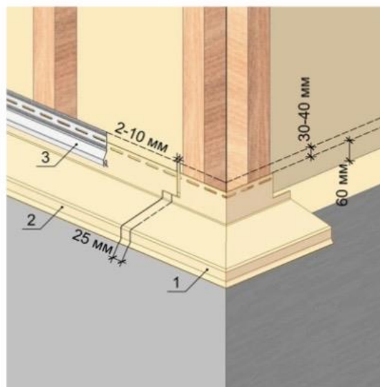
Рис. 5 Установка пластикового отлива Döcke.
