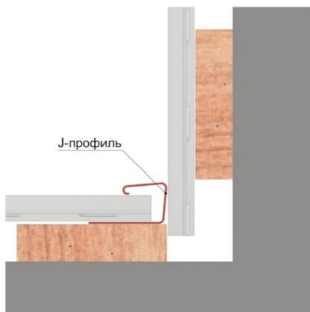
Рис. 16 Монтаж обрешётки под внутренний угол
