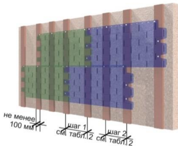
Рис. 4 Вертикальная обрешётка под фасадные панели Döcke BERG и ДЮФУР (для фасадных панелей ДЮФУР шаг 1 меньше, чем шаг 2)
