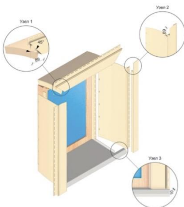
Рис. 15 Обрамление оконного проёма при помощи наличника 89 мм с откосом 254 мм.
