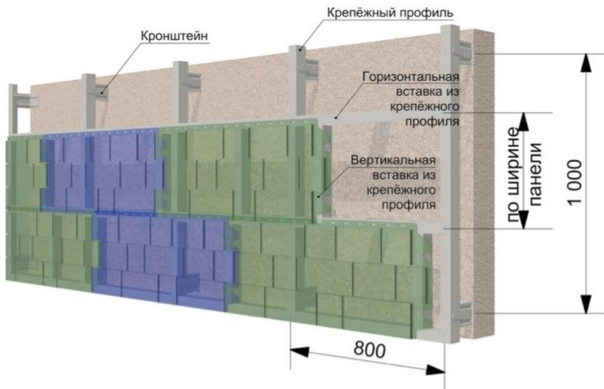
Рис. 8 Установка вертикальных вставок
