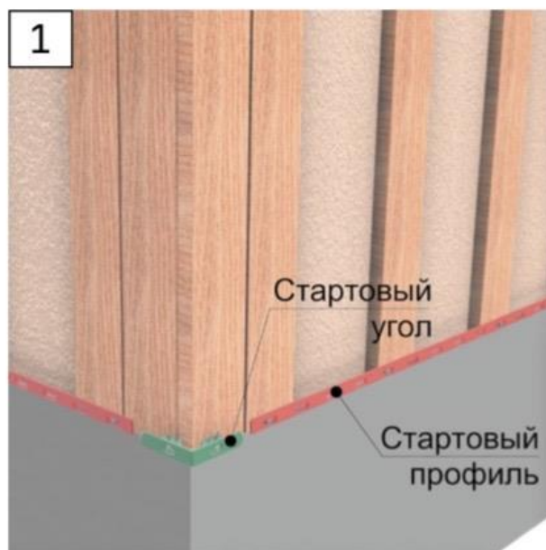
Рис. 9 Установка стартовых профилей и стартовых углов
