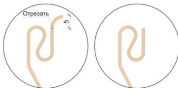
Рис. 10 Подрезка стартового профиля для сайдинга под дерево.
