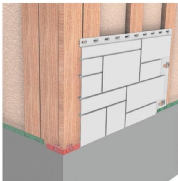
Рис. 18 Монтаж первой панели
