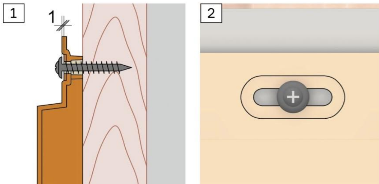
Рис. 2 Схема фиксации фасадных панелей Döcke
