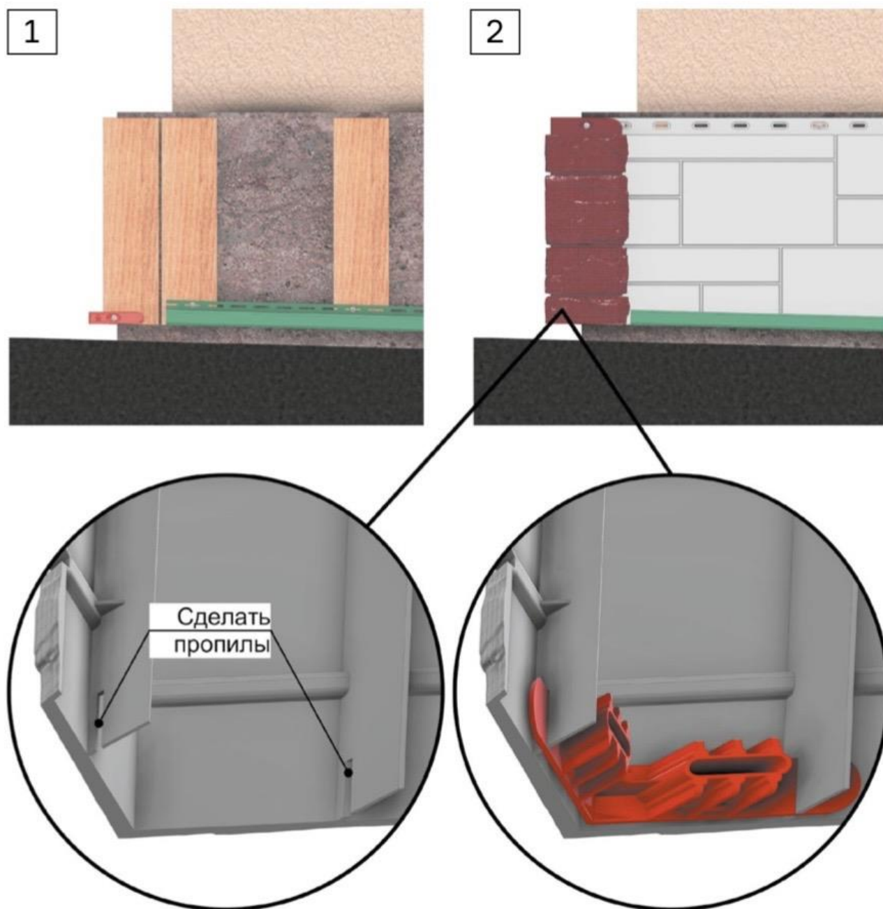
Рис. 21 Отделка цоколя с перепадом высоты
