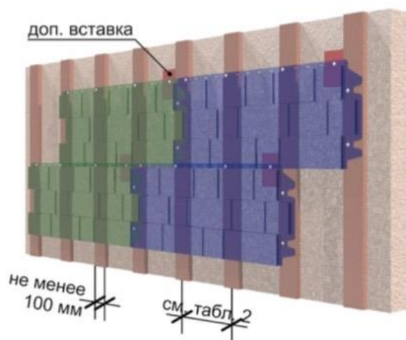
Рис. 5 Вертикальная обрешётка под фасадные панели Döcke FELS и BURG
