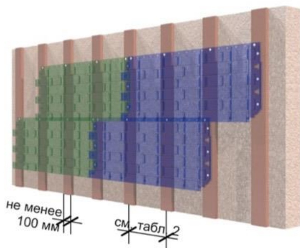
Рис. 3 Вертикальная обрешётка под фасадные панели Döcke ФЛЕМИШ, KLINKER, STERN, СЛАНЕЦ
