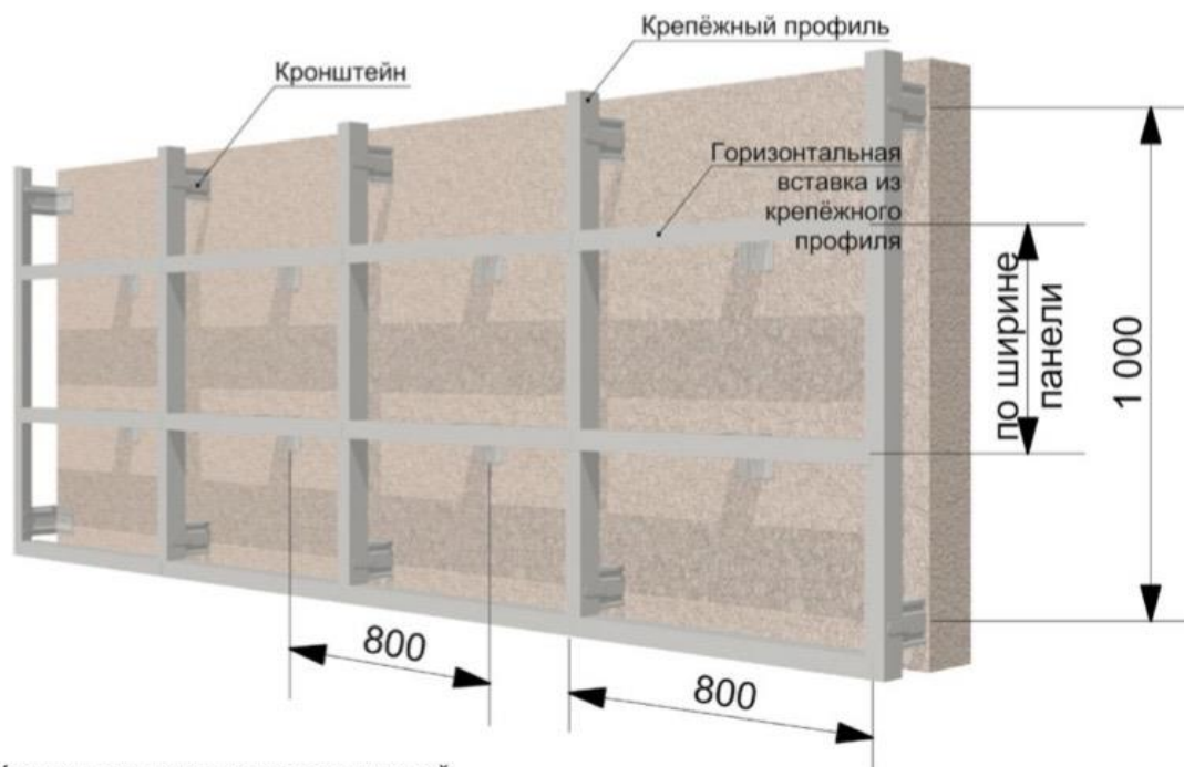
Рис. 7 Установка основания металлической обрешётки под фасадные панели Döcke (вертикальные вставки не показаны (см. рис. 8))
