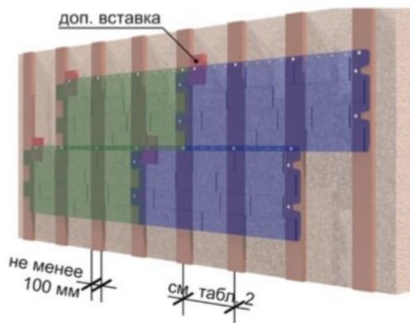
Рис. 6 Вертикальная обрешётка под фасадные панели Döcke STEIN и АЛТАЙ
