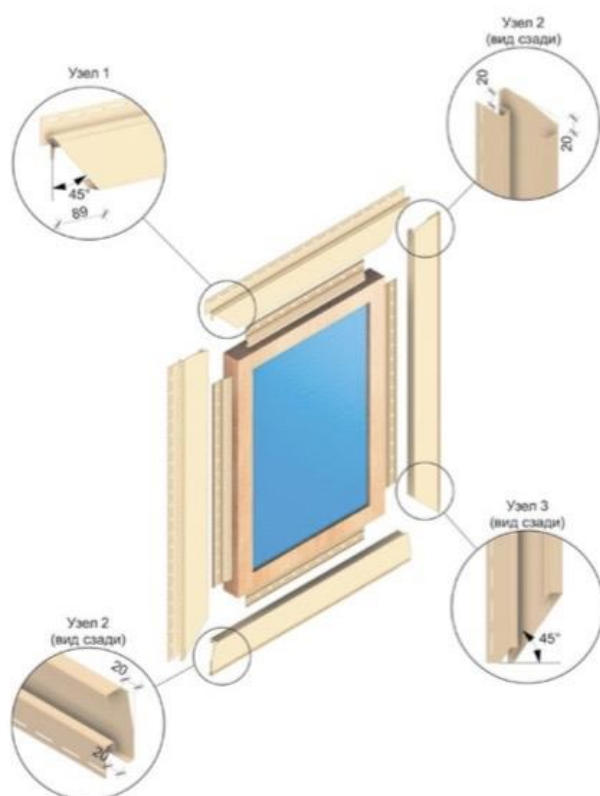
Рис. 11 Обрамление оконного проёма при помощи наличника 89/30 мм.
