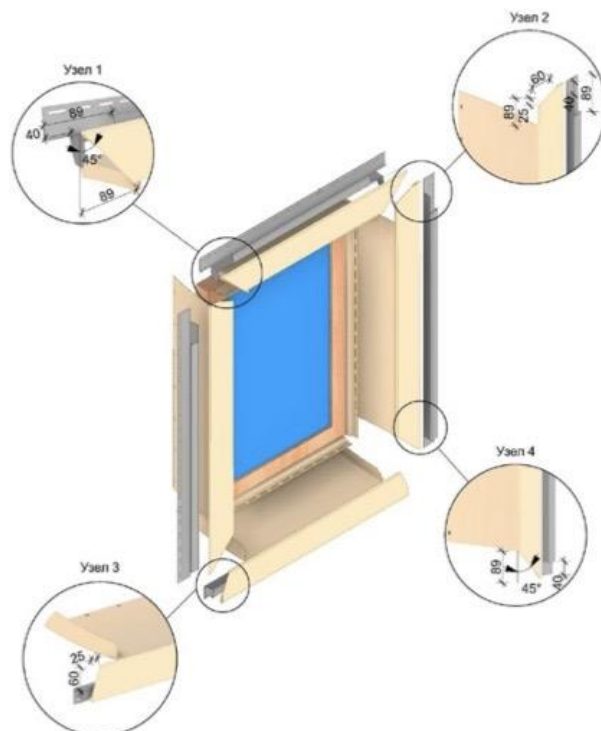
Рис. 13 Обрамление оконного проёма при универсального околооконного профиля с соответствующим J-профилем (таблица 4).
