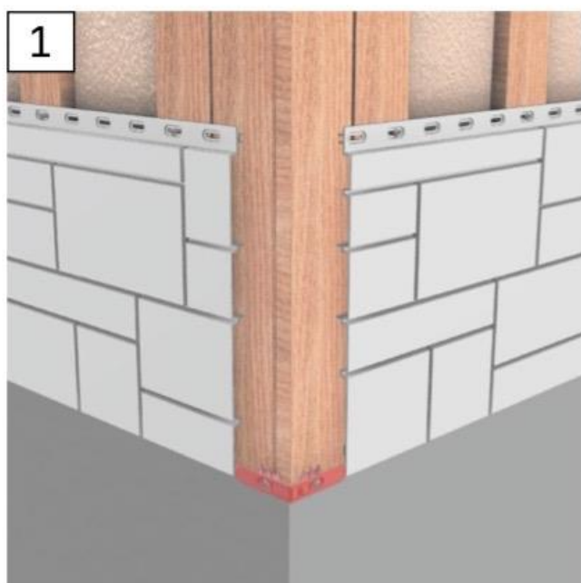
Рис. 19 Монтаж первого ряда панелей
