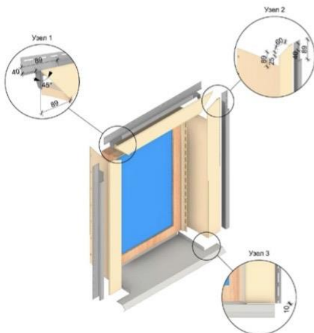
Рис. 14 Обрамление оконного проёма при универсального околонного профиля с соответствующим J-профилем (таблица 4) при наличии металлического отлива.
