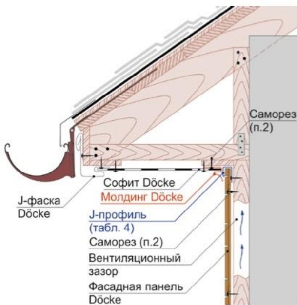
Рис. 22 Примыкание фасадных панелей Döcke к карнизному свесу.
