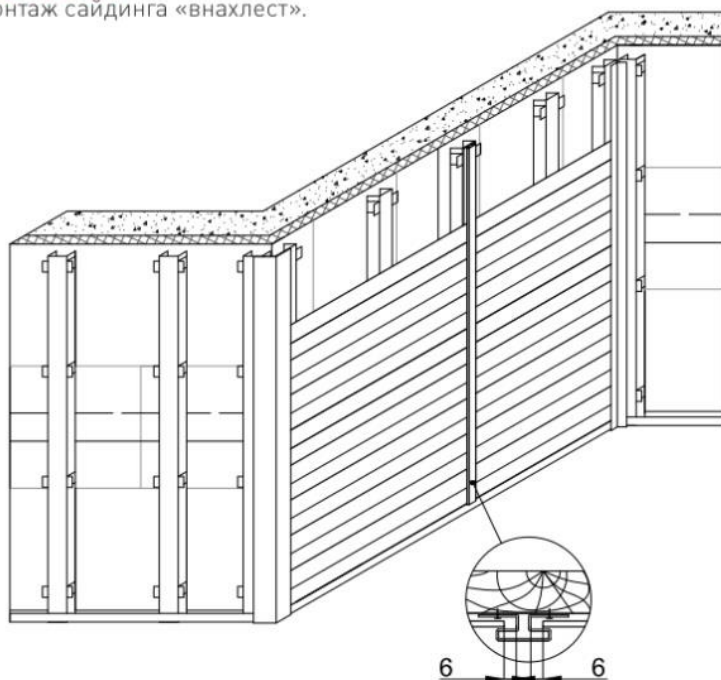
РИСУНОК 7а Монтаж сайдинга «внахлест».
